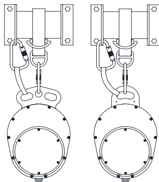
МОНТАЖ С ОДНОЙ ТОЧКОЙ МОНТАЖА (предпочтительный вариант)
