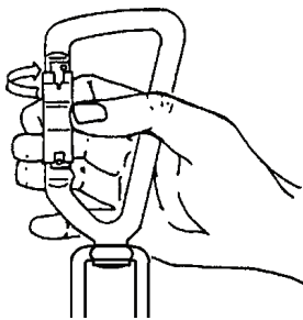
б) Поверните муфту карабина на 90 градусов вокруг своей оси
