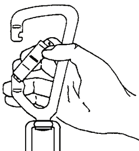
б) Нажимайте на муфту, пока она не повернется вокруг защелки
