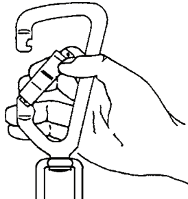
с) Нажимайте на муфту, пока она не повернется вокруг защелки
