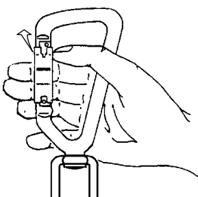
а) Поднимите муфту карабина до упора
