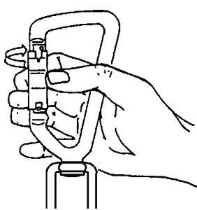
а) Поверните муфту карабина на 90 градусов вокруг своей оси
